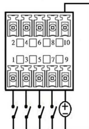
Digital Input Wiring
